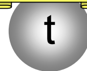
top-Quark
