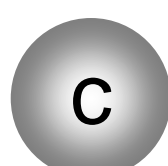
charm-Quark
