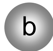
bottom-Quark
