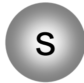
strange-Quark
