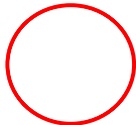
strange-Quark
