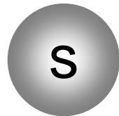
strange-Quark
