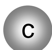
charm-Quark
