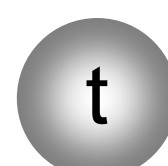
top-Quark
