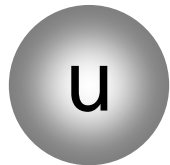
up-Quark
