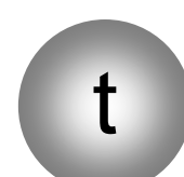
top-Quark
