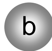
bottom-Quark
